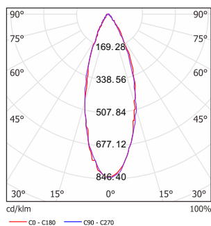
NEVSP30/MR16 7W 24°
