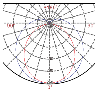
NEVB01 14W 150°
